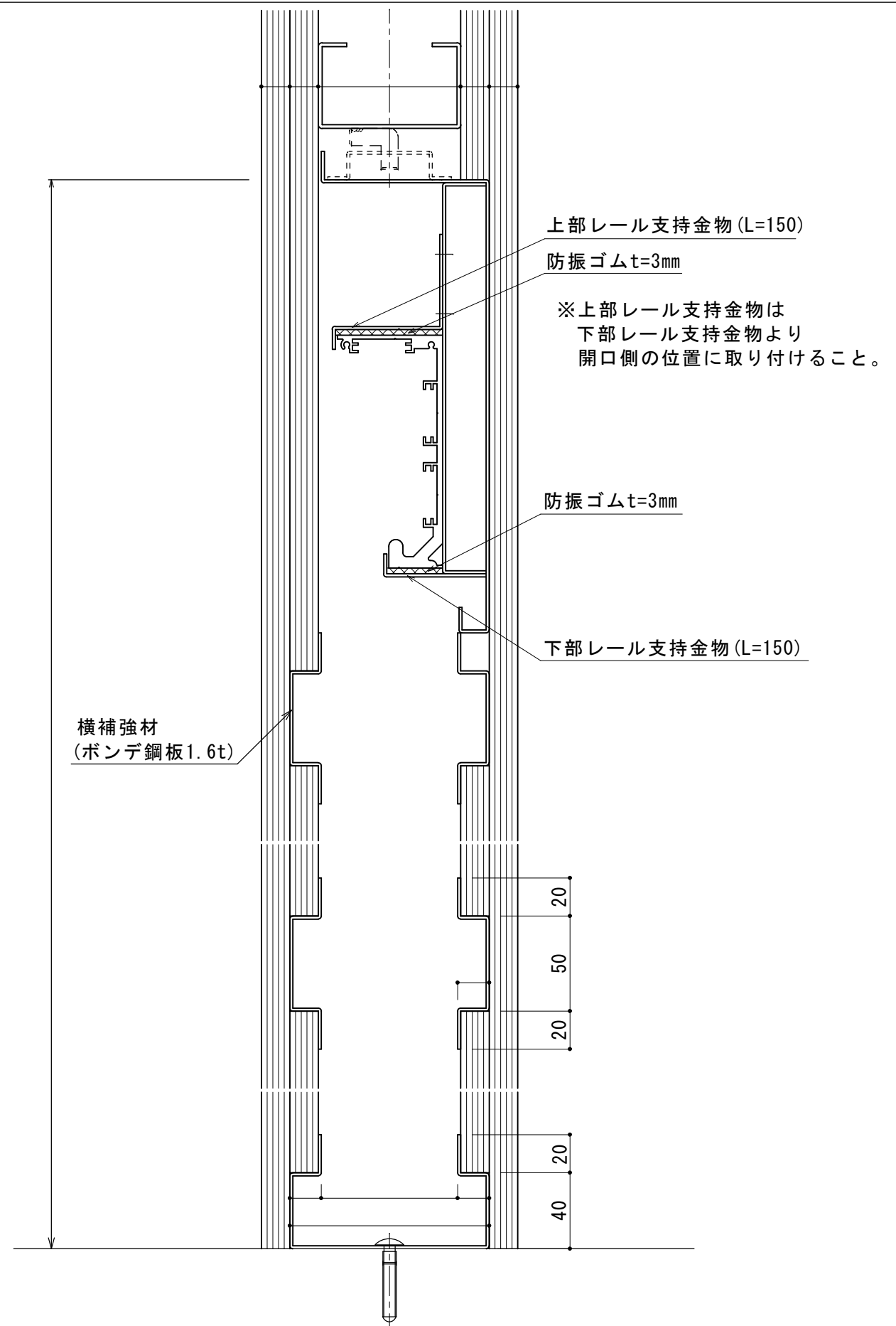
収納壁部縦断面図 S=1/2
