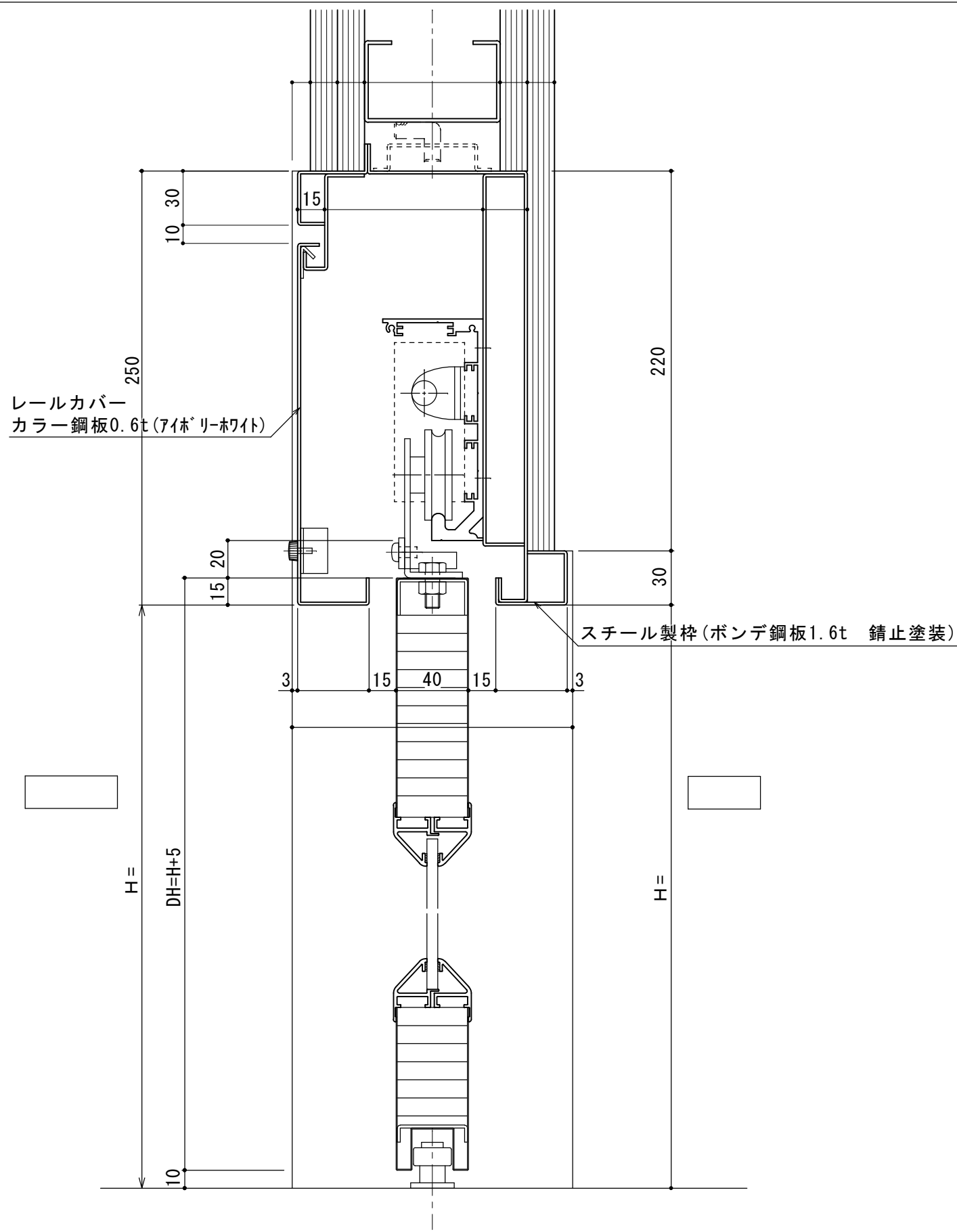
開口部縦断面図 S=1/2
